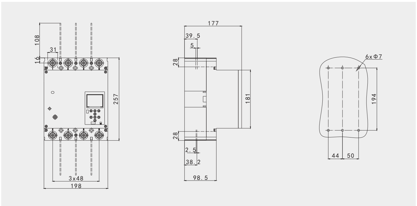
6.2、HYM1LC-400外形及安装尺寸
